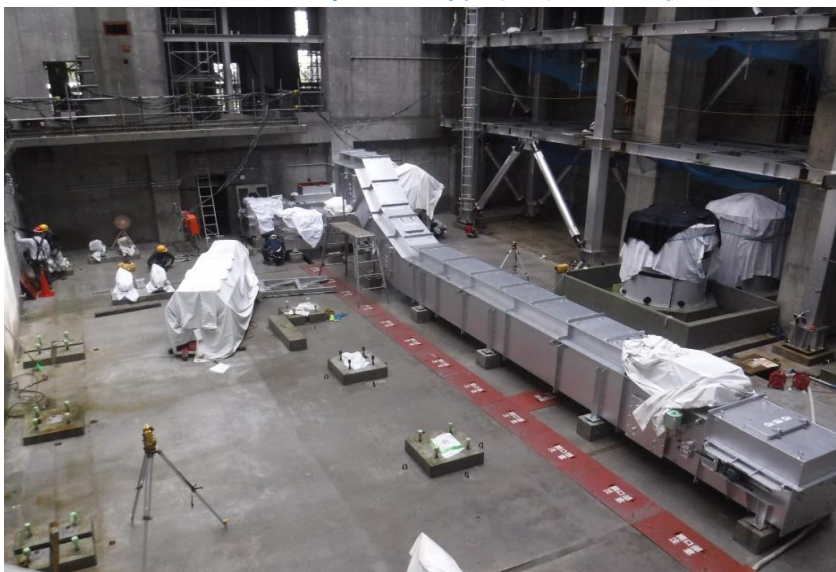
●1工区鉄分搬送コンベヤ取り込み状況
