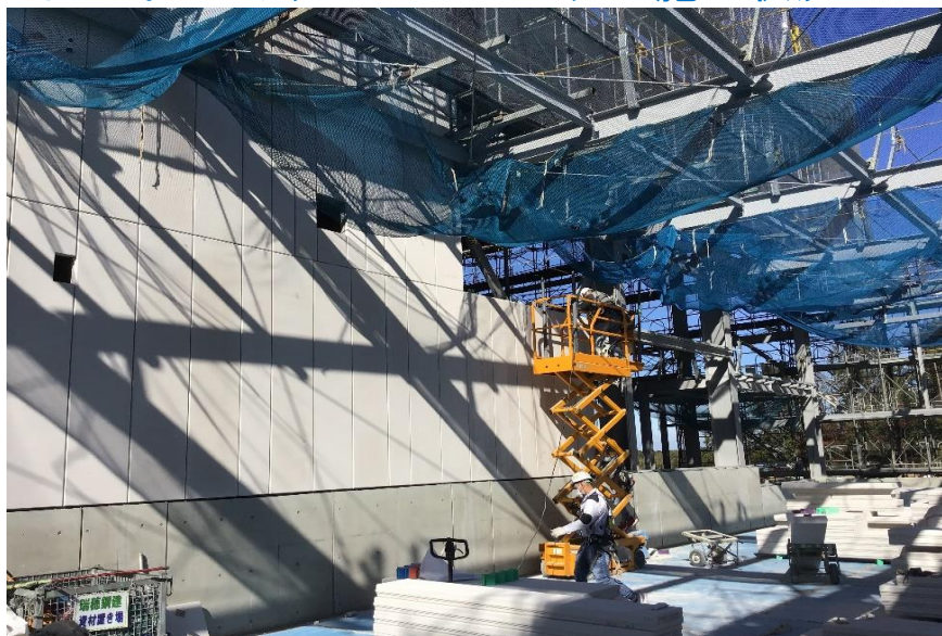
●3工区ストックヤードALC壁施工状況
