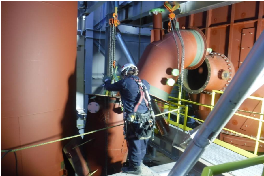
●1工区排ガスダクト組立状況
