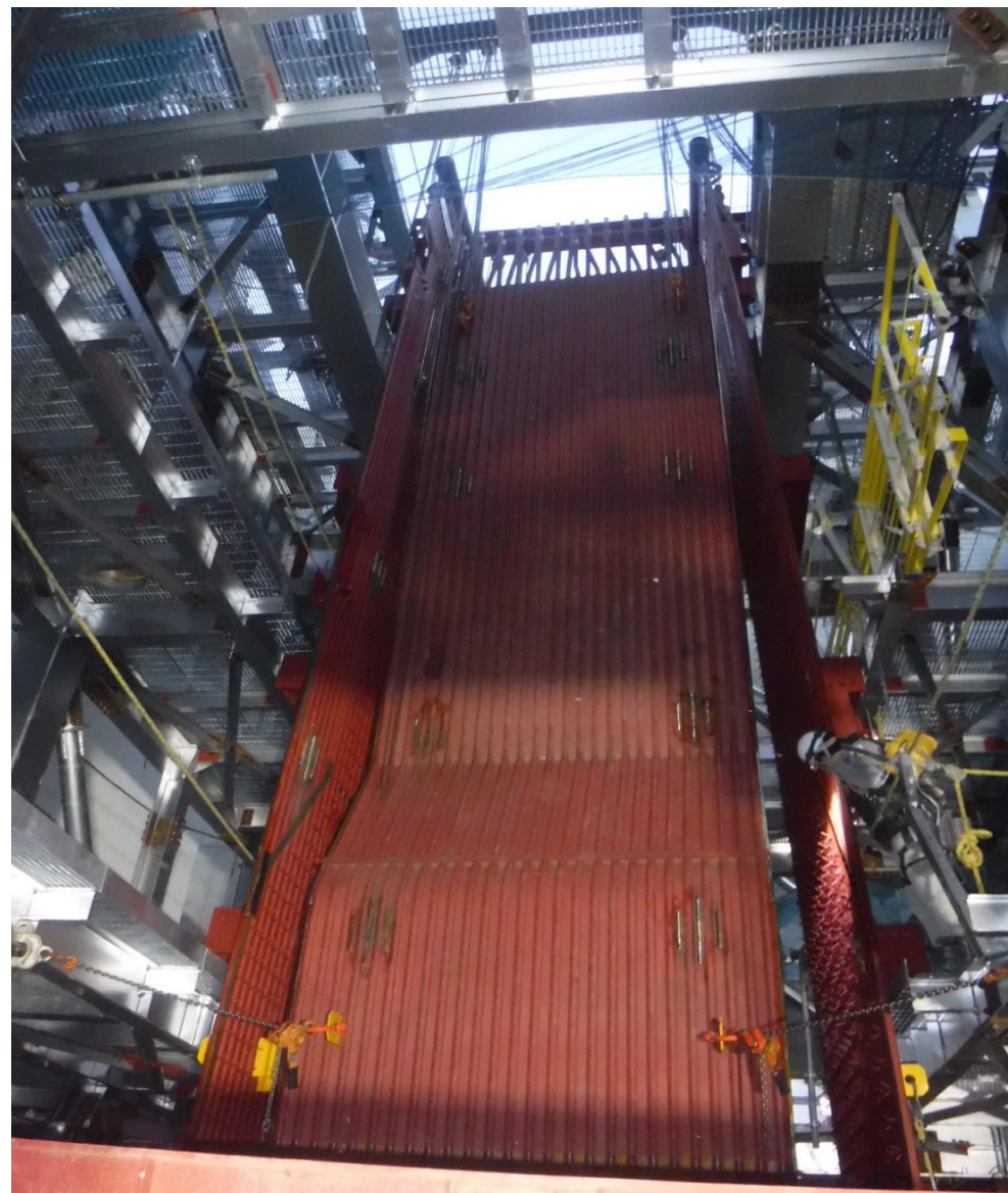
●1工区ボイラ水管壁パネル炉室内取込み状況
