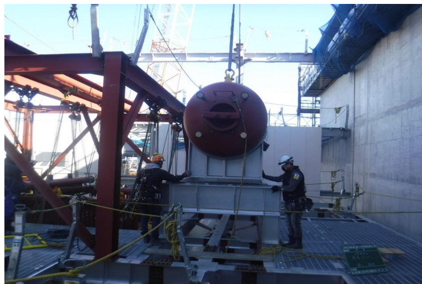
●1工区ボイラドラム据付状況
